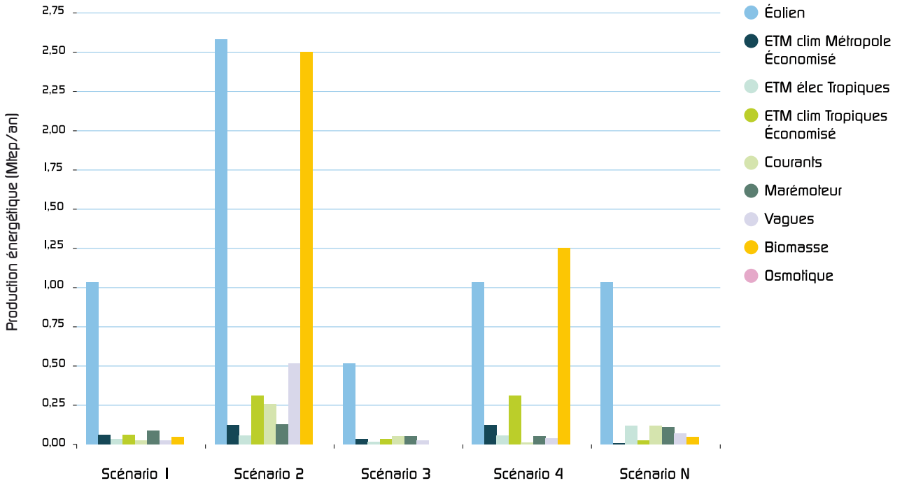
Graph 1 : répartition de la production énergétique des technologies suivant les scénarios (4 scénarios contrastés à 2030 | 1 scénario normalif à 2020 suivant engagement UE) visualisation avec éolien marin
