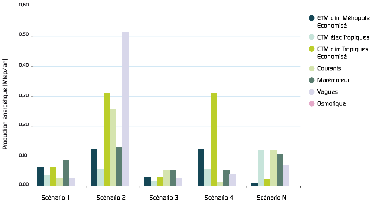
Graph 2 : répartition de la production énergétique des technologies suivant les scénarios (4 scénarios contrastés à 2030 | 1 scénario normalif à 2020 suivant engagement UE) visualisation sans éolien marin ni biomasse
